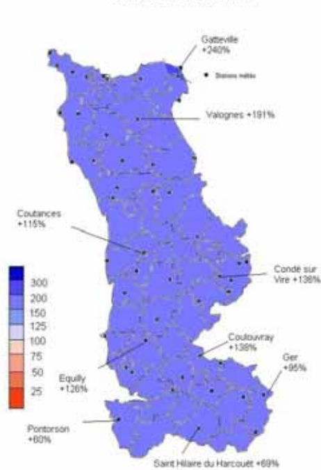
PLUVIOMETRIE NOVEMBRE 2009 ECART A LA MOYENNE
